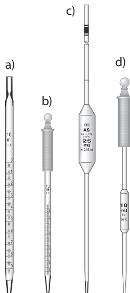
Fig. 7.2. Pipete pentru măsurarea volumului soluțiilor: a – pipetă gradată; b – pipetă gradată cu piston; c – pipetă cotată cu bulă; d – pipetă cotată cu piston
