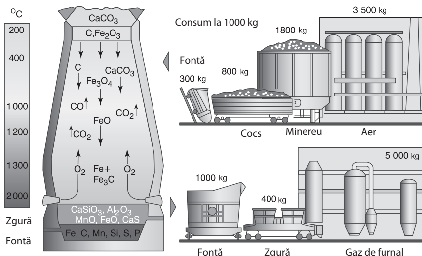
Fig. 4.4. Schema producerii fontei
