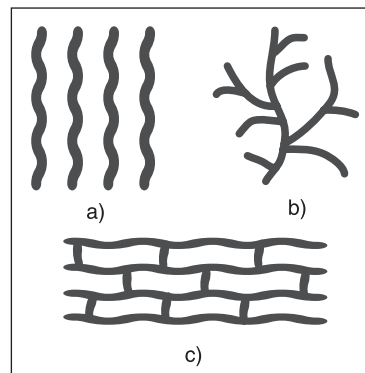
Fig. 2.14. Formele geometrice ale macromoleculelor de polimer: a) liniare; b) ramificate; c) reticulate
