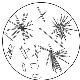
Fig. 6.1. Cristale de CaSO_4 \cdot 2H_2O
