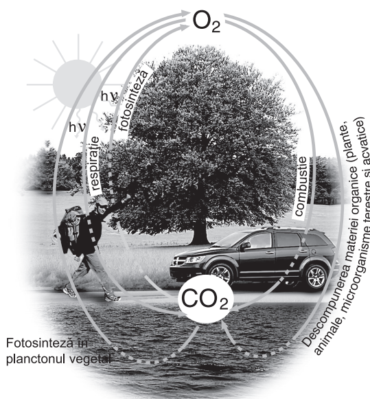
Fig. 2.4. Circuitul oxigenului și al dioxidului de carbon în natură
