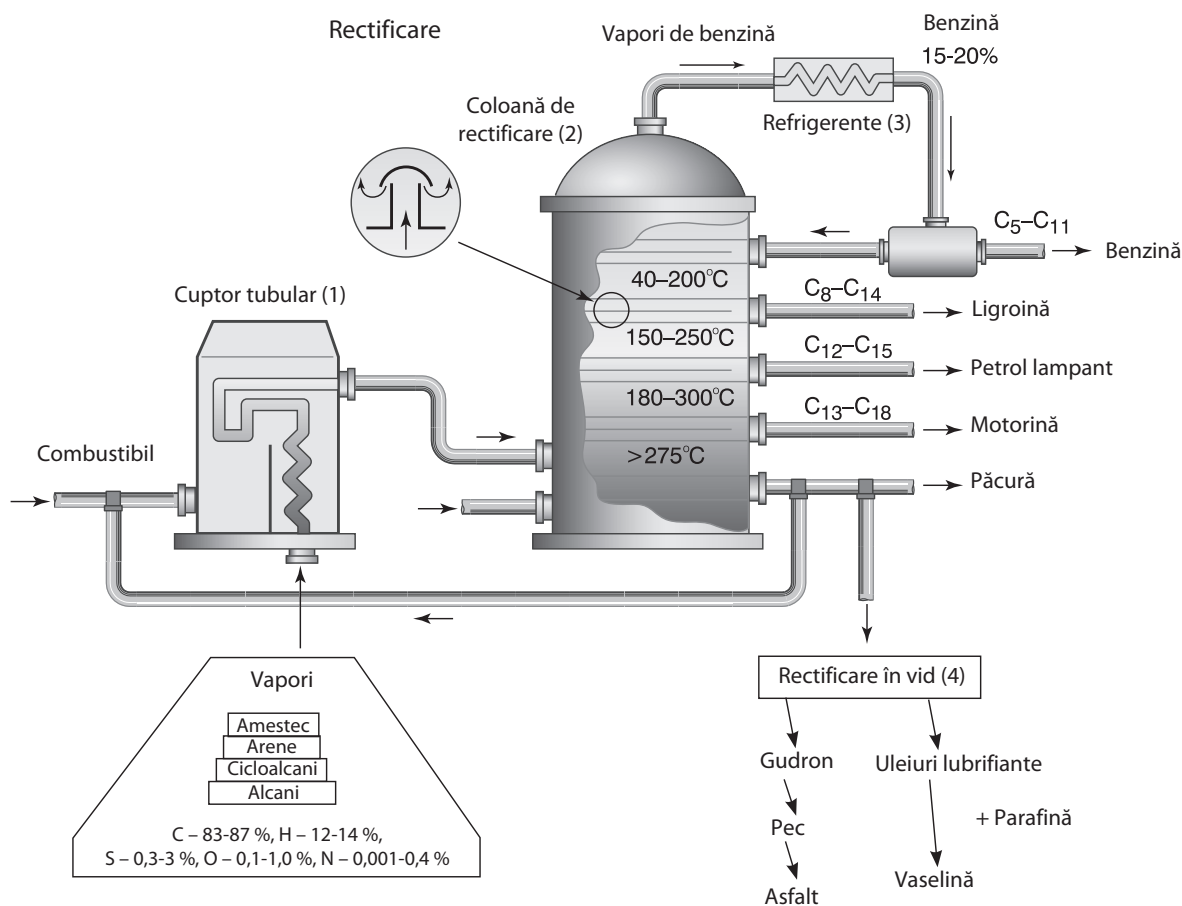
Fig. 4.5. Prelucrarea petrolului (1 – cuptor tubular, 2 – coloană de rectificare, 3 – refrigerent, 4 – rectificare în vid)
